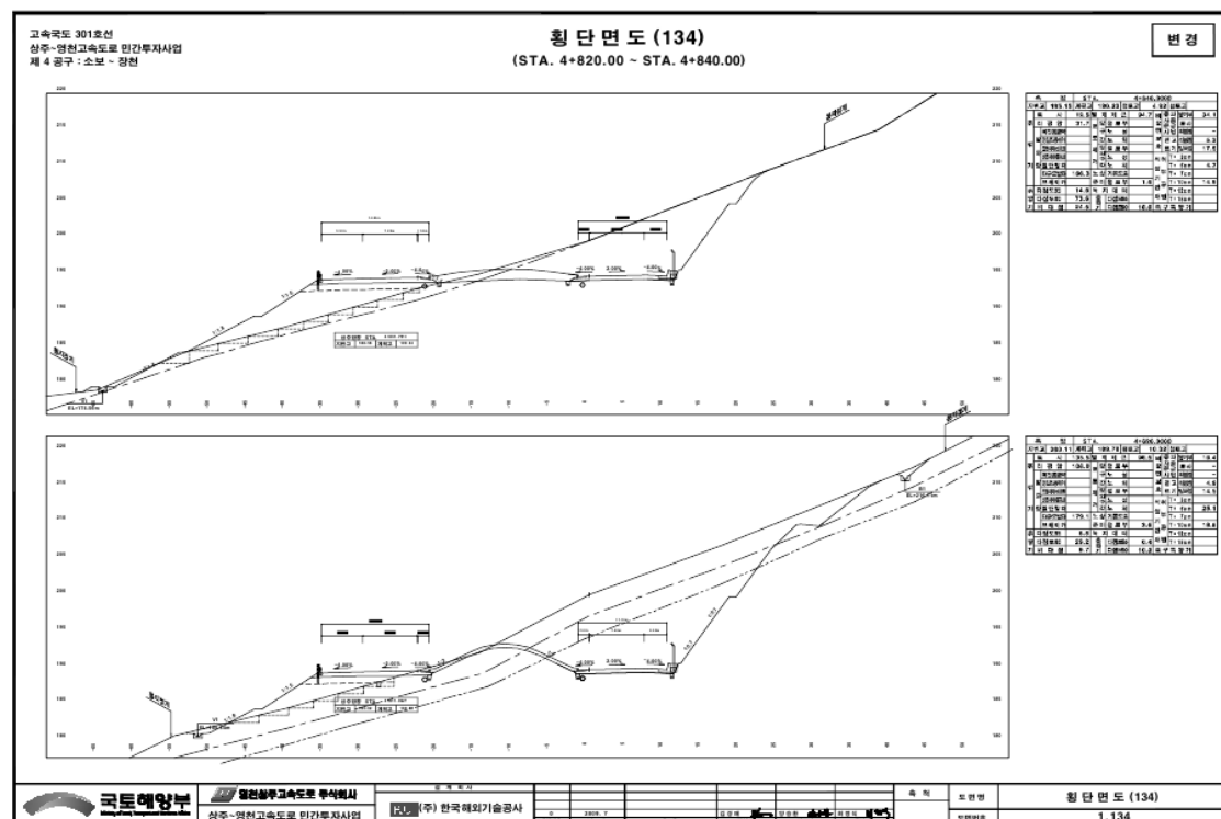
【그림 26.4】 표준횡단면도
